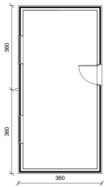
תכנית
