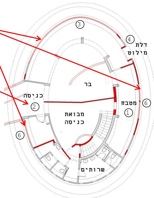
תכנית ק.קרקע, מצב קיים
