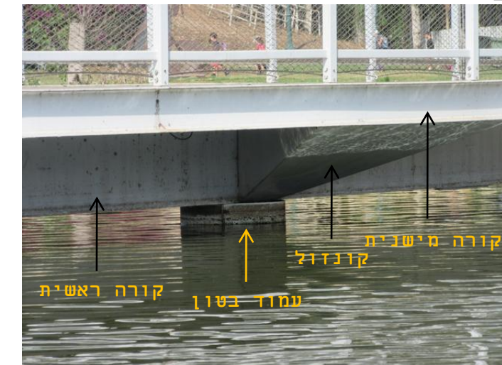
31. עמוד בטון עגול תומך קורת ו מפלדה, ממנה יוצאים שני קונזולות לתמיכת המדרג
