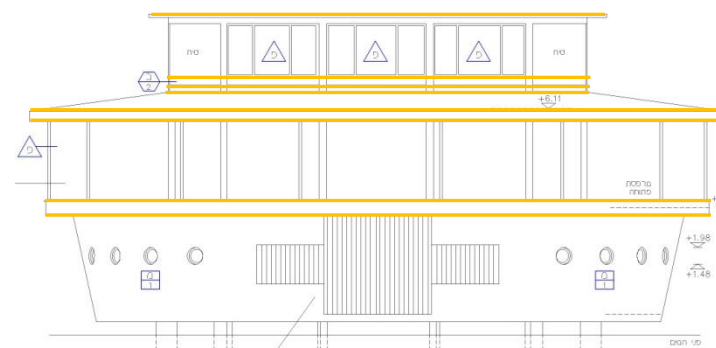
חזית הכניסה המזרחית - מצב מקורי משוחזר
