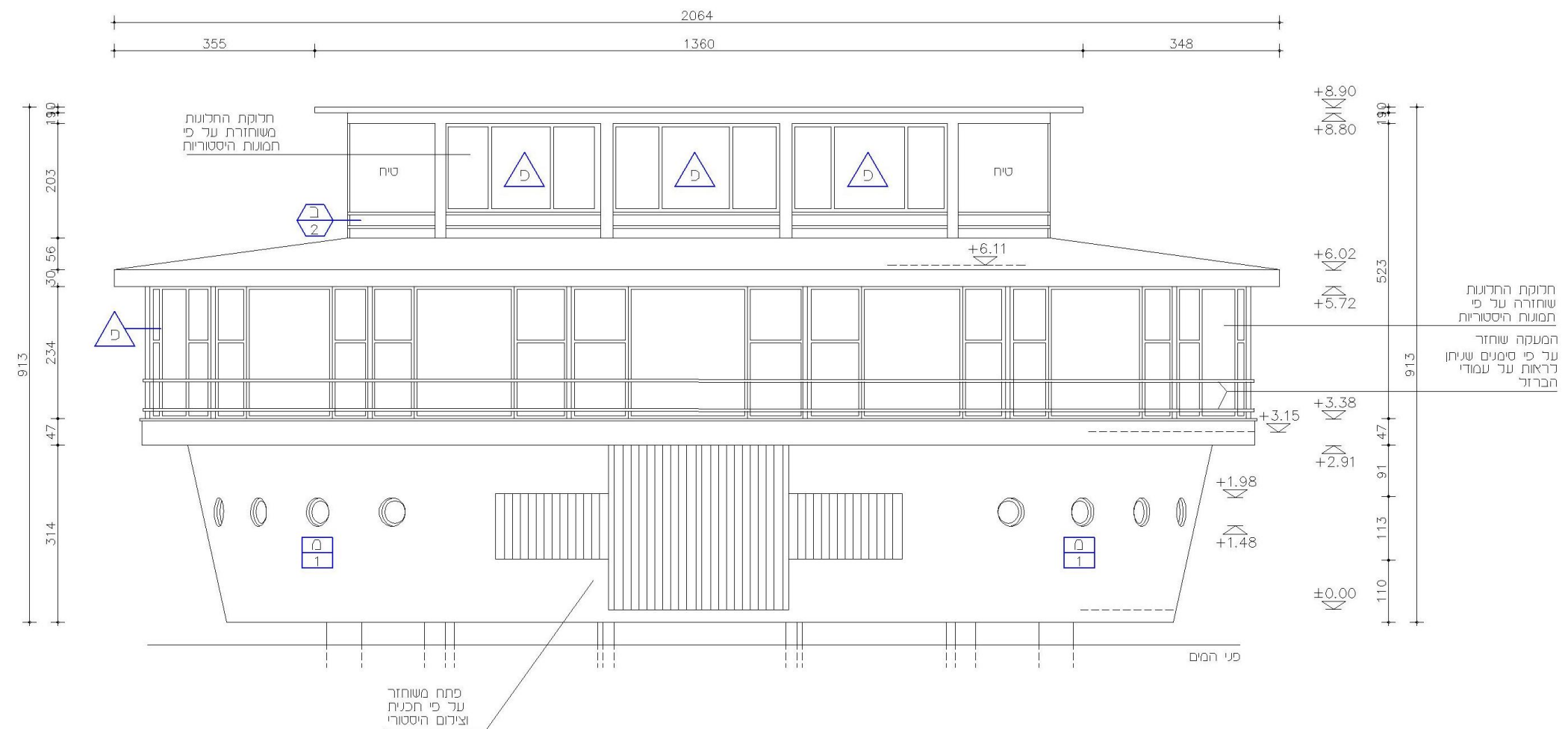
חזית מזרחית - חזית הכניסה המקורית מצב מקורי משוחזר לאחר סגירת קומה א בחלונות בשנת 1967
