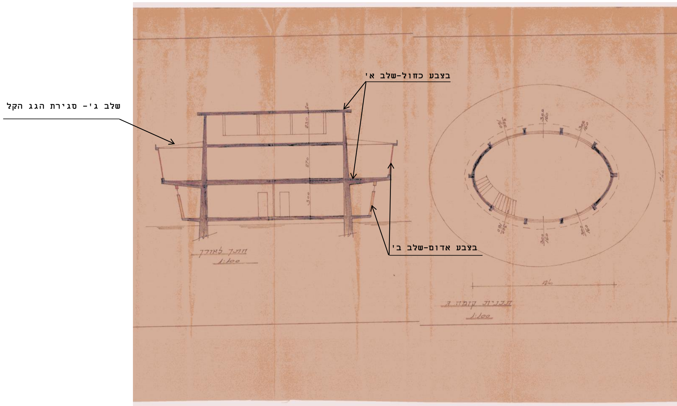
תכנית היסטורית- ניתוח שלבי הבניה
