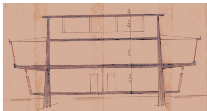
חתך - 1967 קירות קומה ב' תוכננו כאלכסוניים אך נבנו אנכיים.
