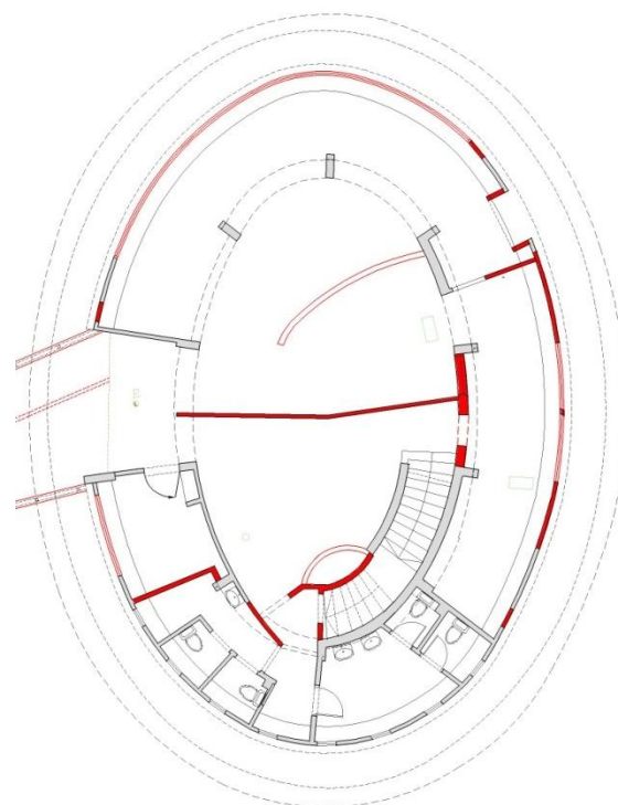
תכנית קומת קרקע מצב קיים
