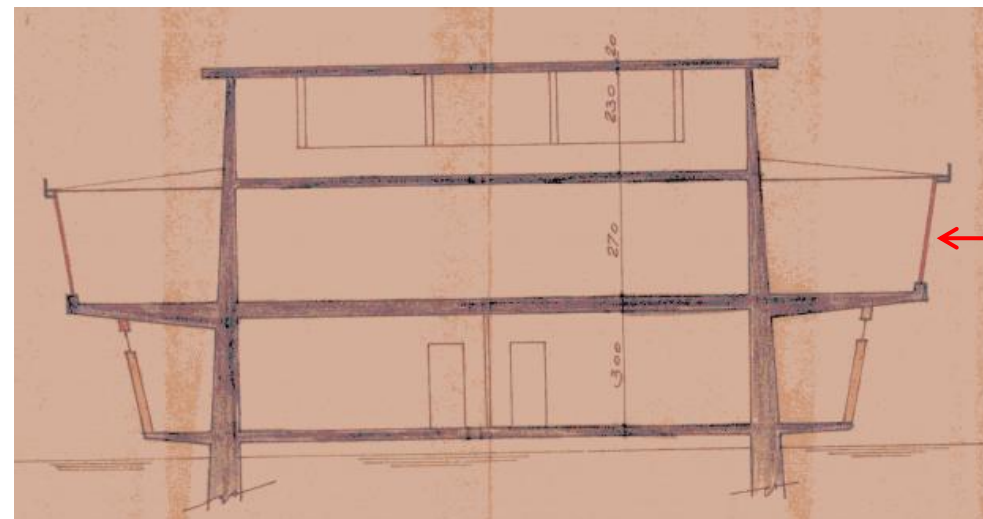
חתך מתוך ההיתר לסגירת המרפסת בקומה א 1967
