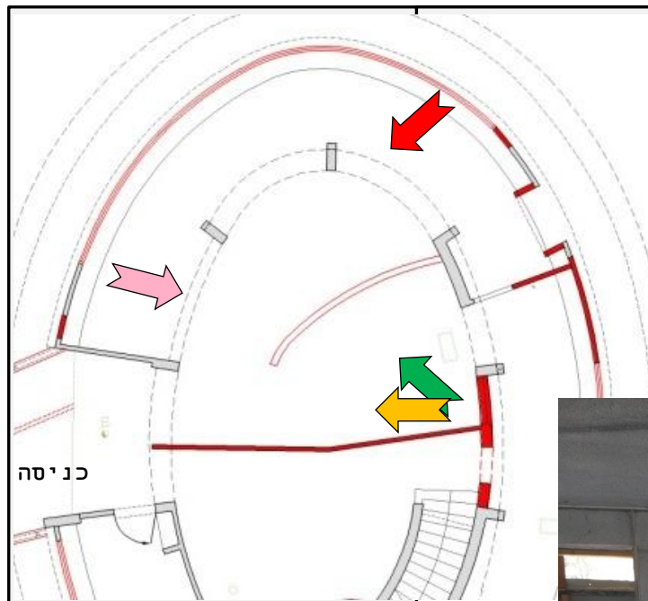
תכנית קומת קרקע
