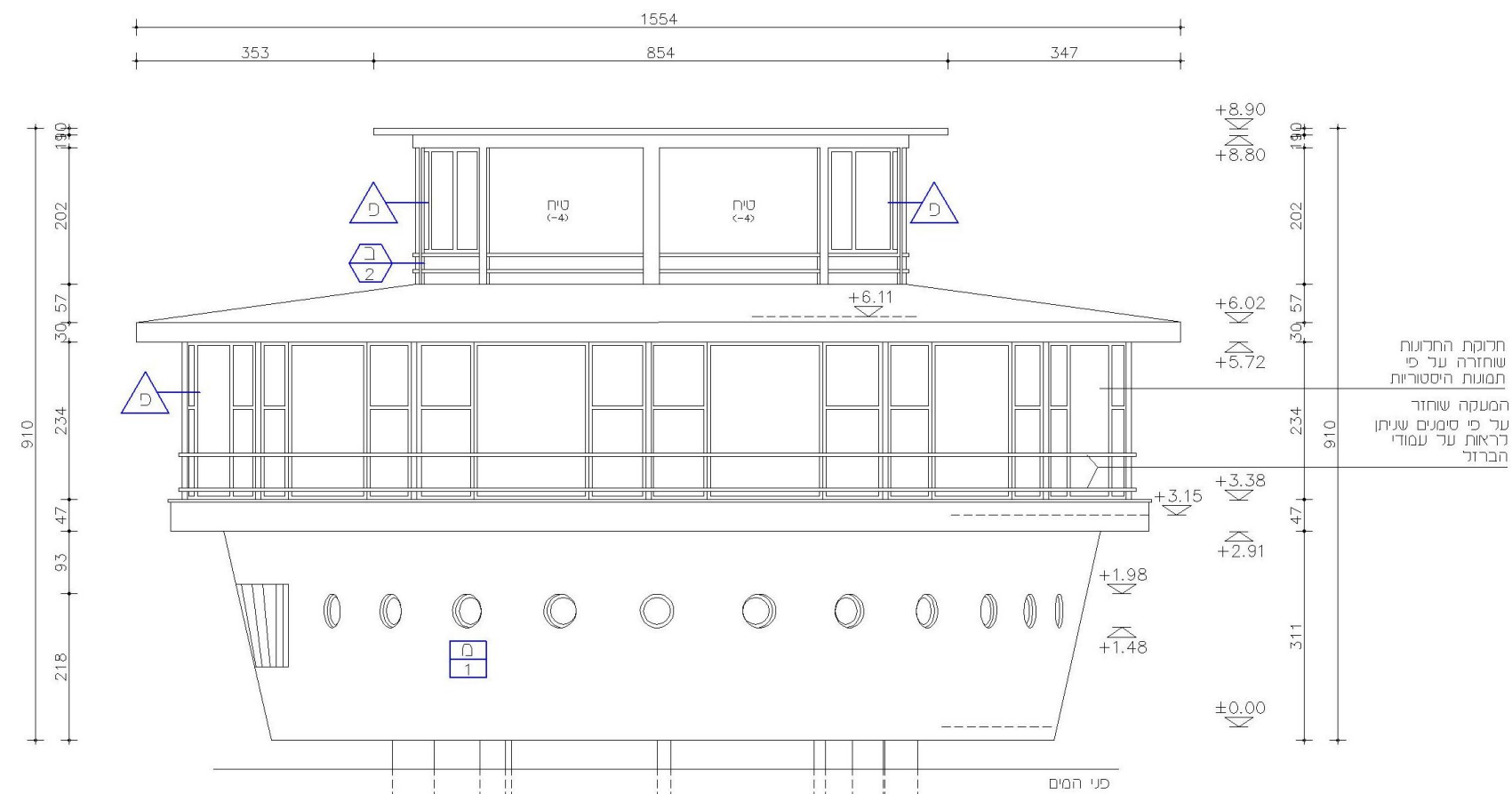
חזית צפונית מצב מקורי משוחזר לאחר סגירת קומה א בחלונות בשנת 1967
