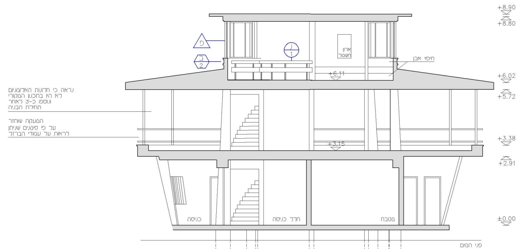
חתך ב-ב מצב מקורי משוחזר
