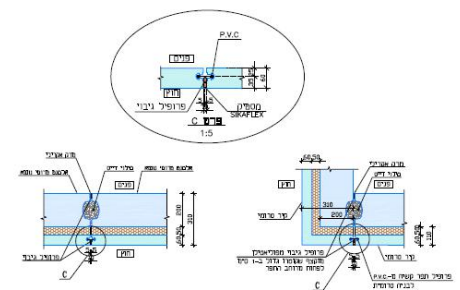
פרט 3 פרט איטום תפר אנכי בין שני קירות טרומיים
