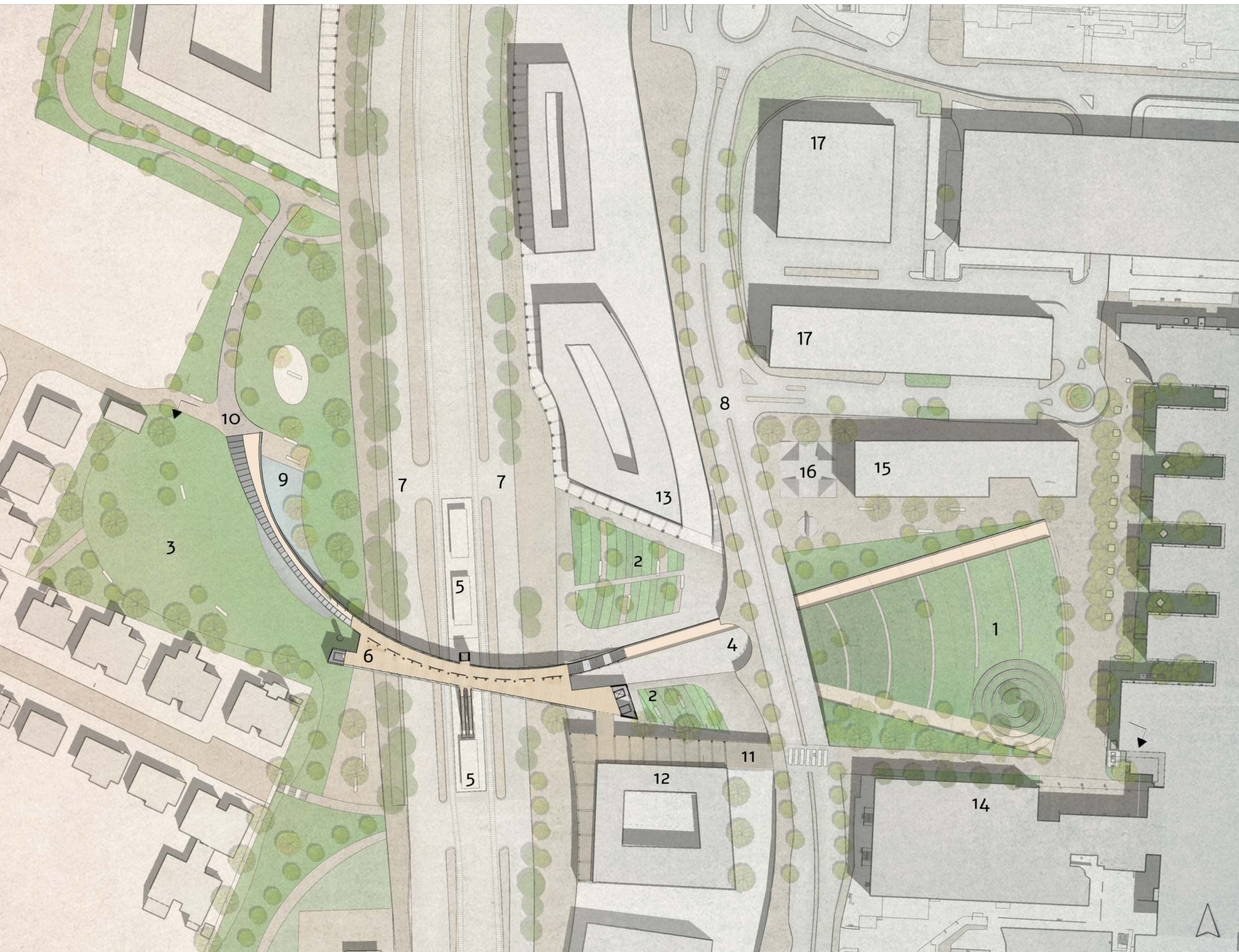
תכנית במפלס הגשר +52.00
