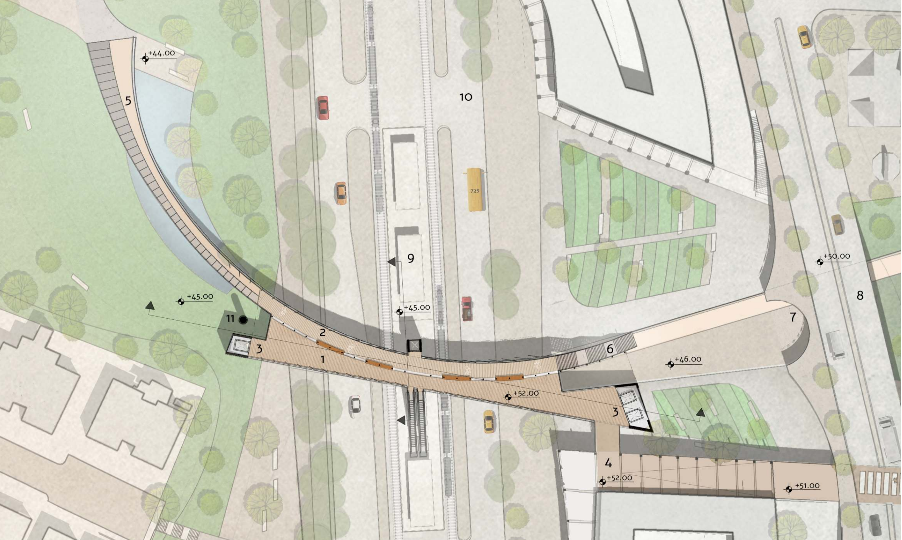
תכנית במפלס הגשר +52.00 הגשר דו תכליתי: מוביל לשער הכניסה החדש, מהשצ"פ המערבי ומתחנת "שיבא מערב" ובמקביל מתחבר למעבר המוצל שמוביל למגדל האשפוז
