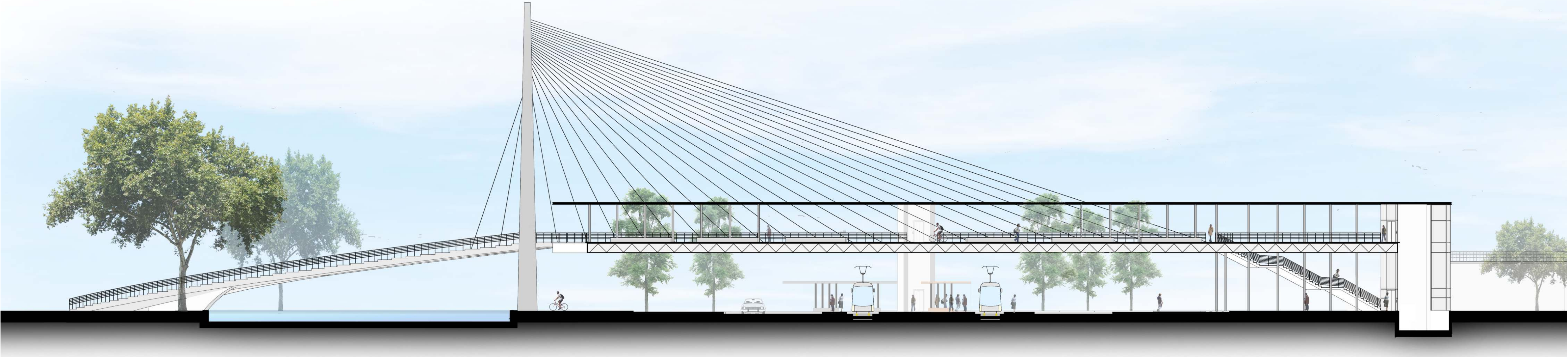
חתך לאורך גשר המיתרים ותחנת הרכבת "שיבא מערב" עם מבט לעבר המדרגה הנופית ורמפת האופניים, הדרגנועים והמעליות המובילים למפלס הגשר
